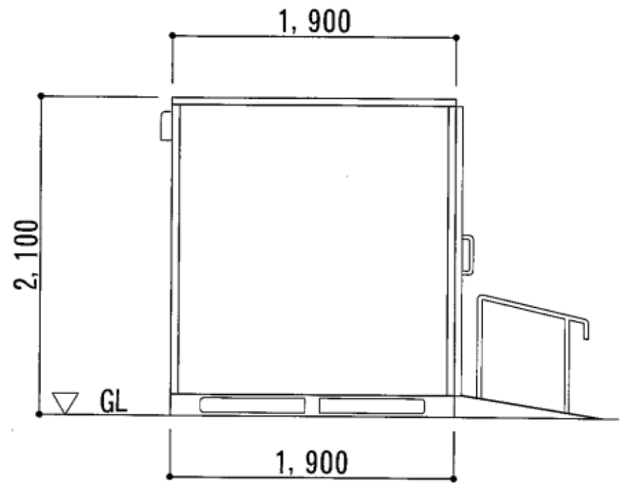
左側面図
