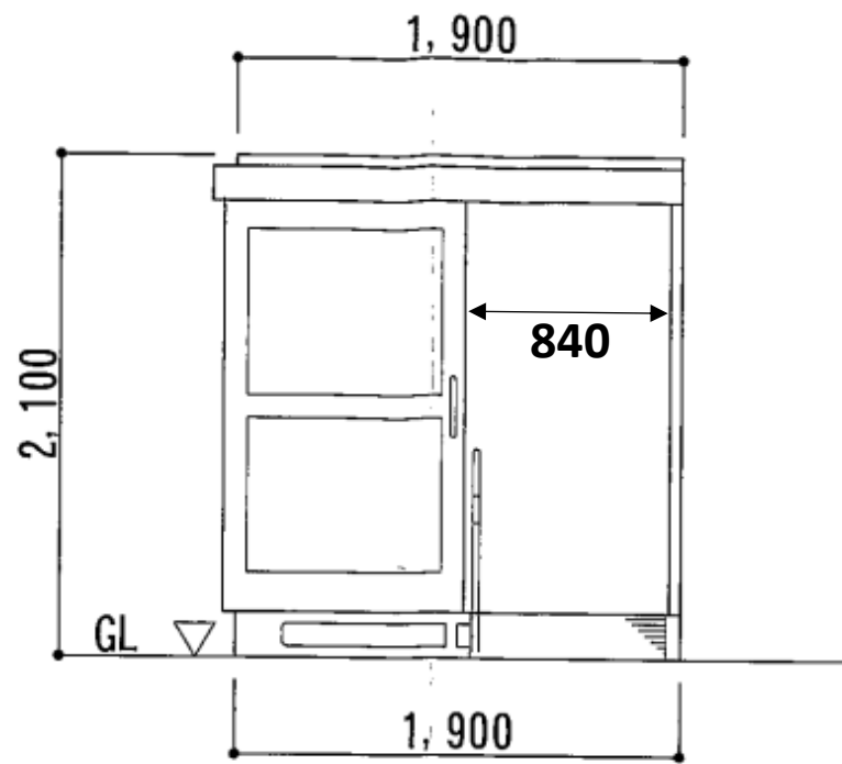
正面図
