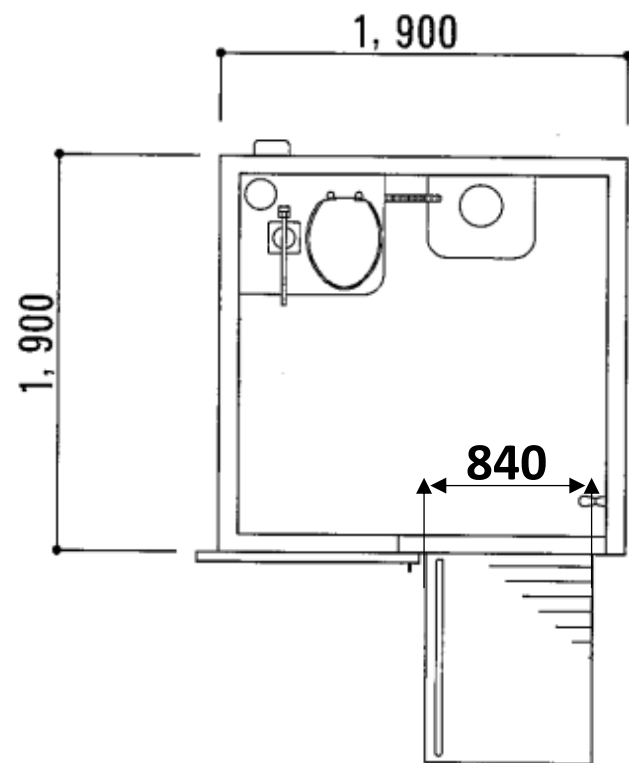
平面図
