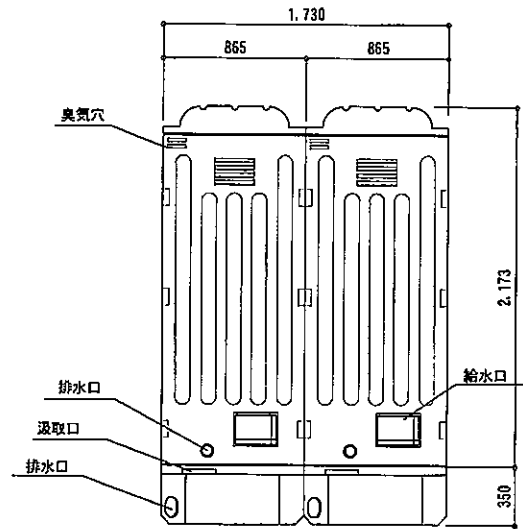
裏面図
