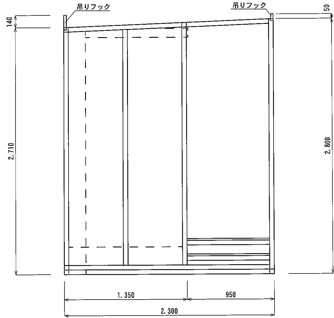
側面図
