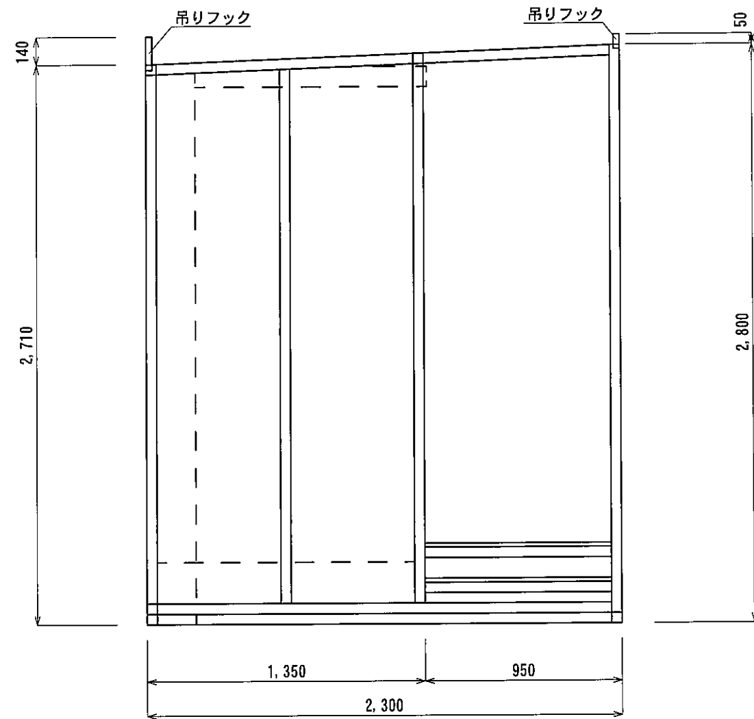
側面図
