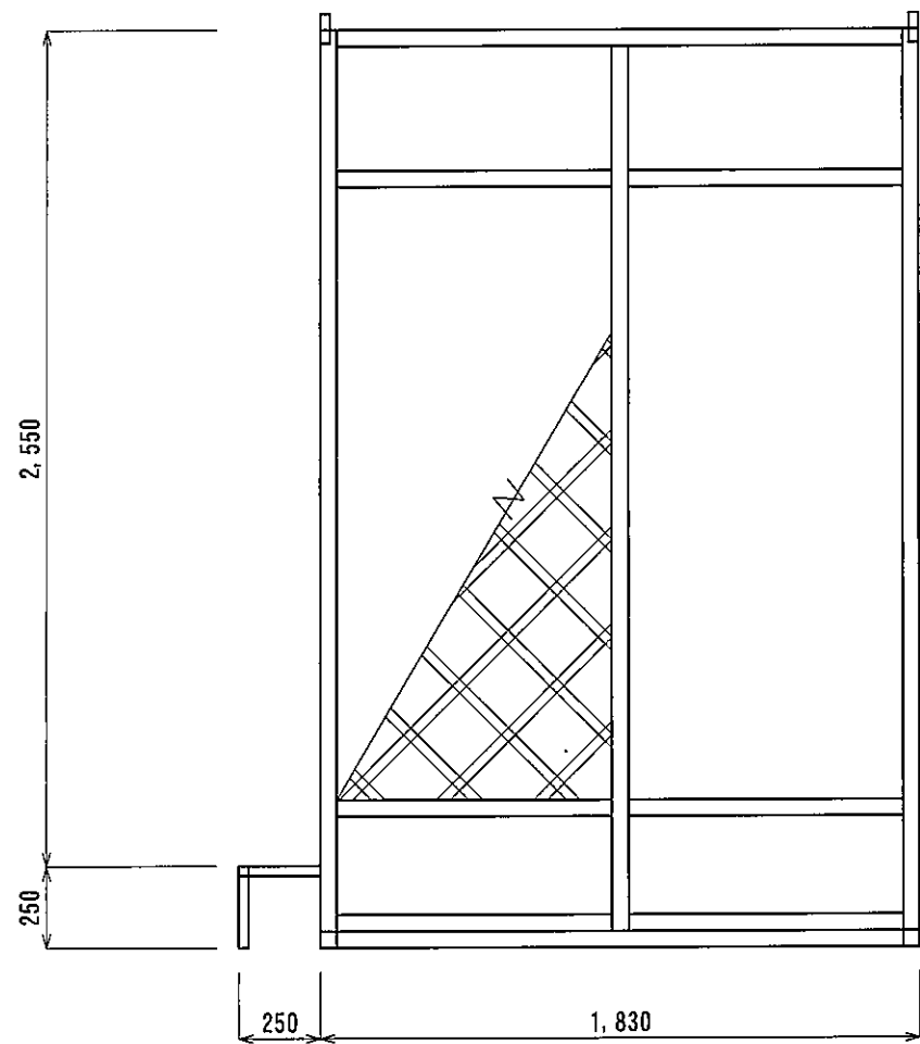
正面図
