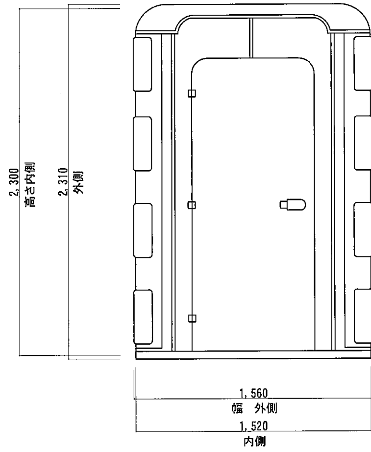
正面図 S=1/30
